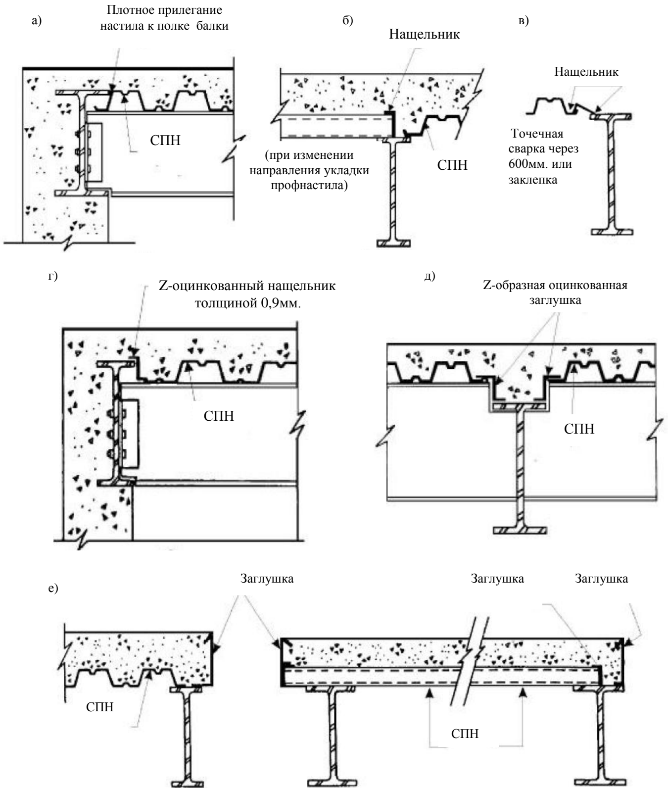
Рис. 5.7 Схемы закрытия технологических отверстий СБП
