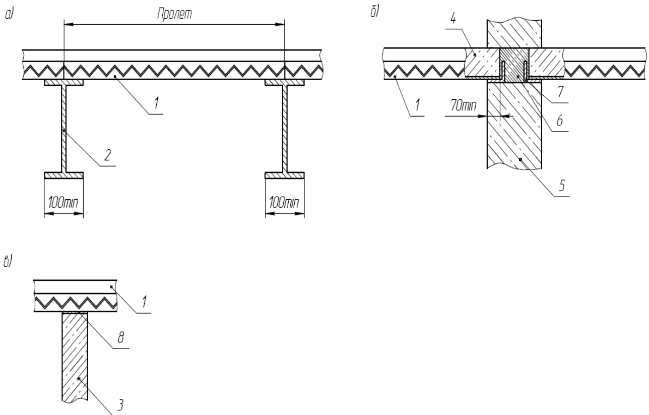
Рис. 5.1 Схемы опирания плиты СБП
