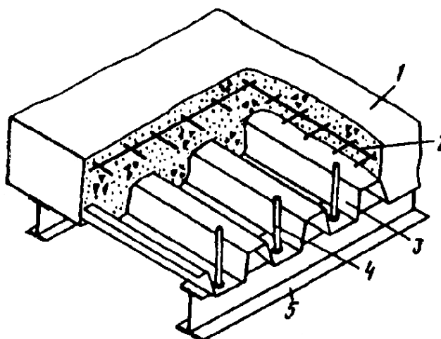
Рис. 5.3 Конструкция СБП
