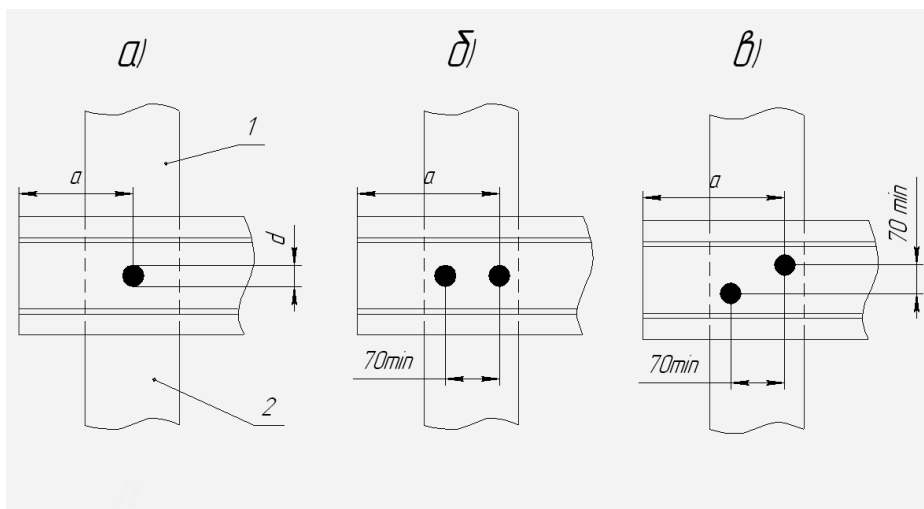
Рис. 5.4 Схемы анкерки
